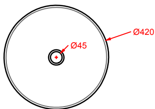
GIL002 GIÒ EVOLUTION lavabo tondo appoggio Ø 42 round countertop washbasin Ø 42
