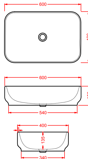
GIL001 GIÒ EVOLUTION lavabo rettangolare appoggio rectangular countertop washbasin
