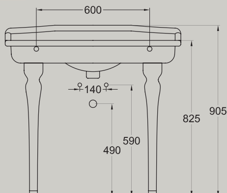
Gamba D35 per consolle D31 Leg D35 for D31
