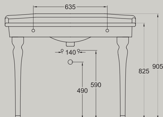
Gamba D35 per consolle D30 Leg D35 for D30
